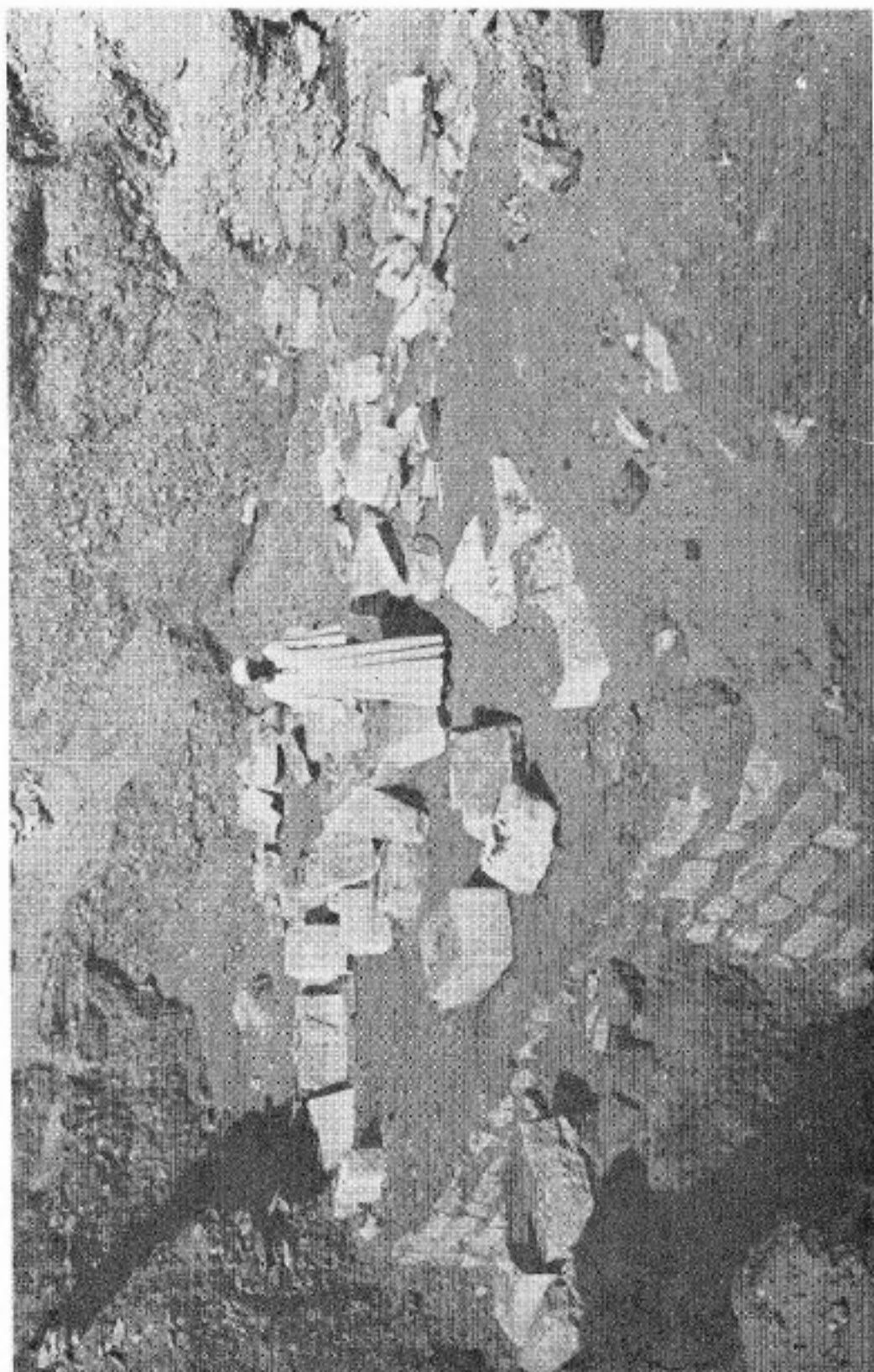
Fondations de la première enceinte de la pyramide de Sekhem-Khet vers le Sud.
